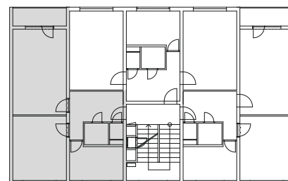
PÔDORYS 5.NP
