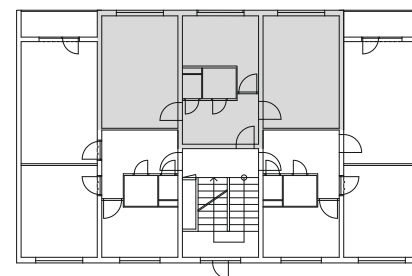
PÔDORYS 1.NP
